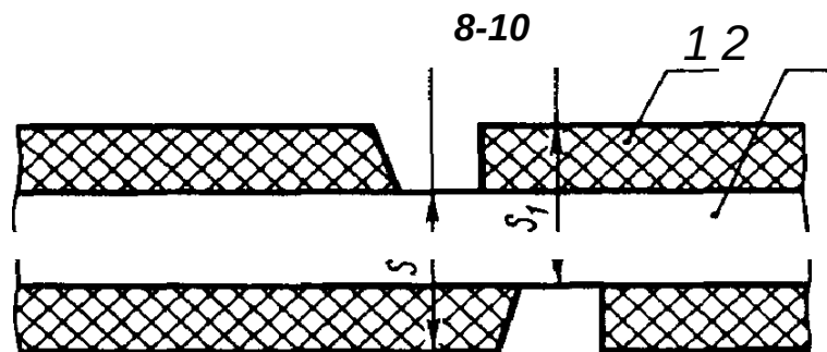
1 — покрытие электрода; 2 — стержень электрода
