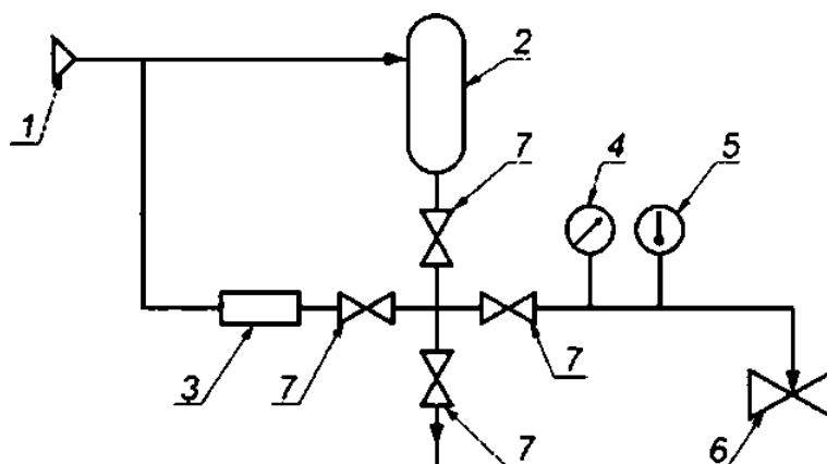
Рисунок Б.7 — Рекомендуемая схема стенда для испытаний обратной арматуры на герметичность затвора и проверку функционирования
