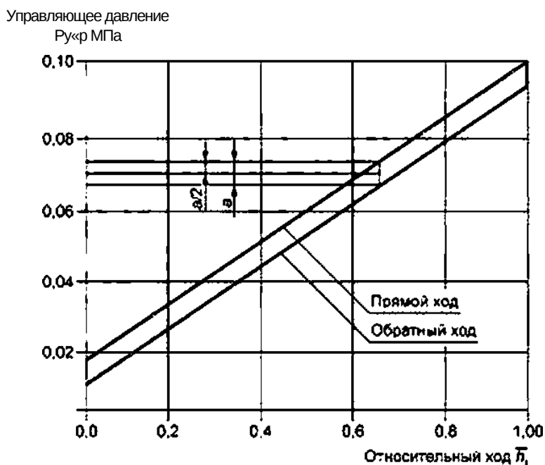
Рисунок 1 — Диаграмма определения нечувствительности регулирующей арматуры «НО» СПИМ для диапазона управляющего давления P_{у.р} от 0,02 до 0,1 МПа
