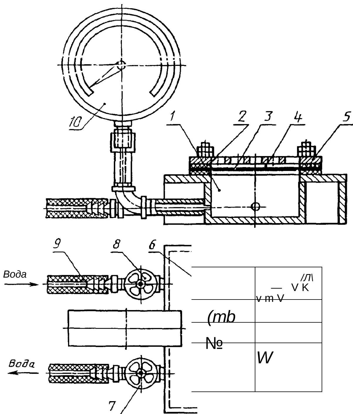
1 — рабочая камера; 2 — резиновые прокладки; 3 — образец; 4 — контактная сегка; 5 — прижимная плита; 6 — зажимные винты; 7, 8 — краны; 9 — резиновая трубка, соединяющаяся с водопроводом; 10 — манометр
