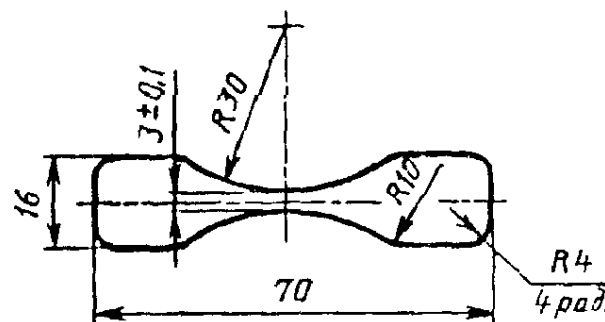
Рисунок 2 — Образец-лопатка типа 2
