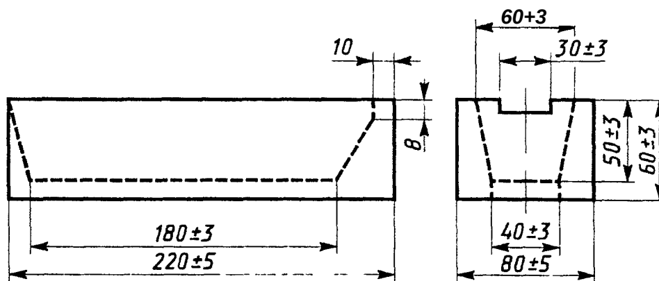
Рисунок 1 — Изложница
