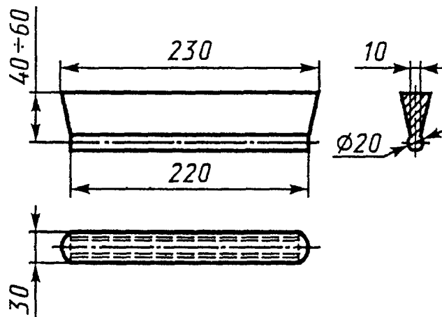
Рисунок 4 — Заготовка для вырезки образцов
